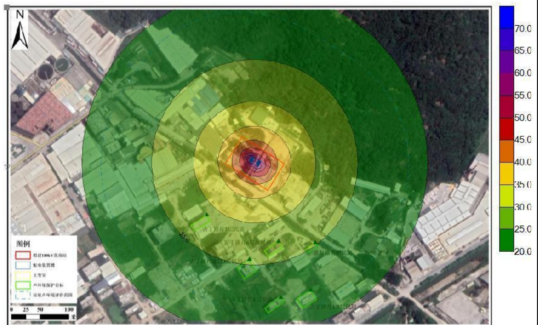
图 4-1 运行期间变电站厂界噪声预测
