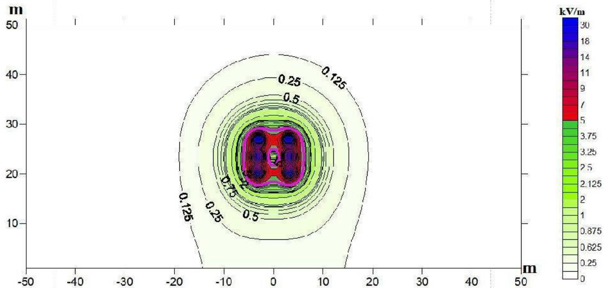
ZT-图 8-5 110kV 双回架空线路工频电场强度预测结果分布断面等值线图
