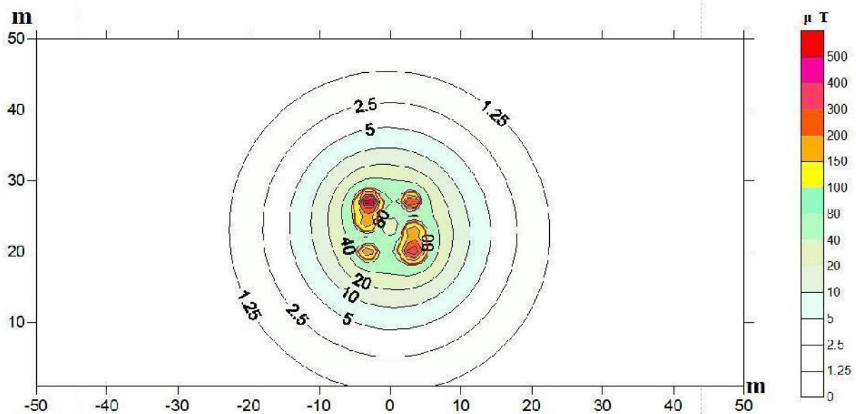
ZT-图 8-7 110kV 双回架空线路工频磁感应强度预测结果分布断面等值线图
