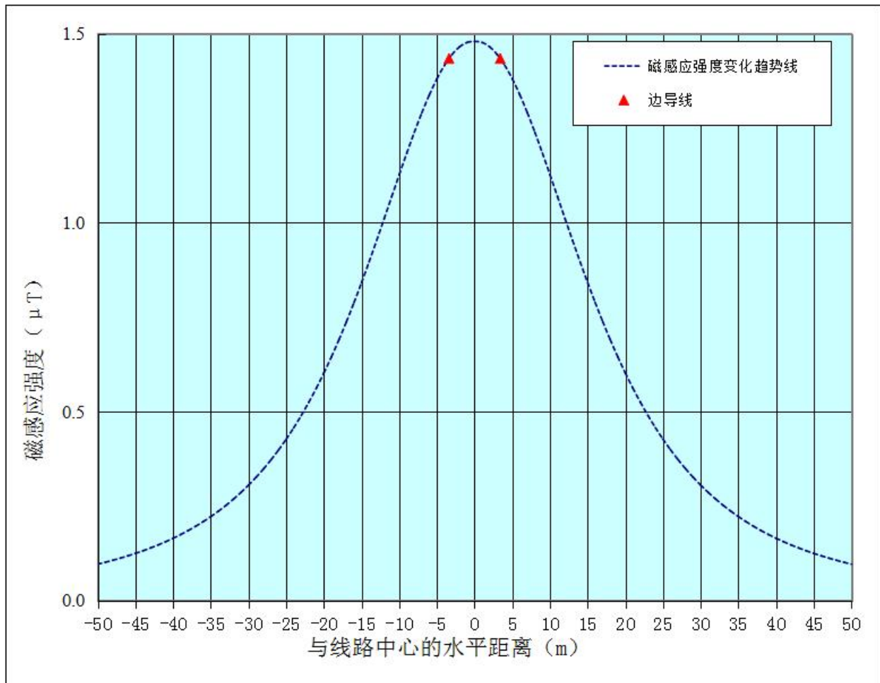
ZT-图 8-6 110kV 双回架空线路工频磁感应强度预测结果衰减趋势线图(离地 1.5m 高处)
