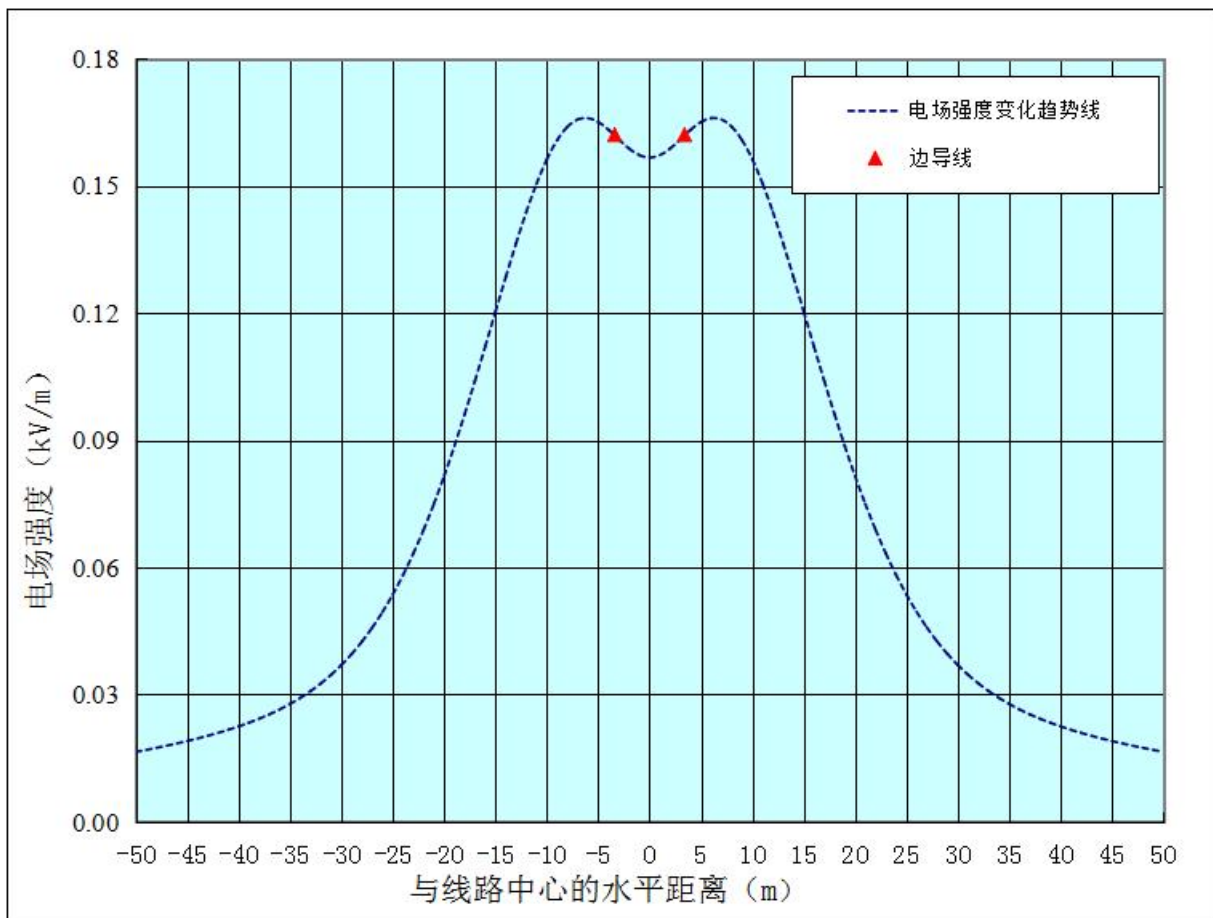
ZT-图 8-4 110kV 双回架空线路工频电场强度预测结果衰减趋势线图（离地 1.5m 高处）
